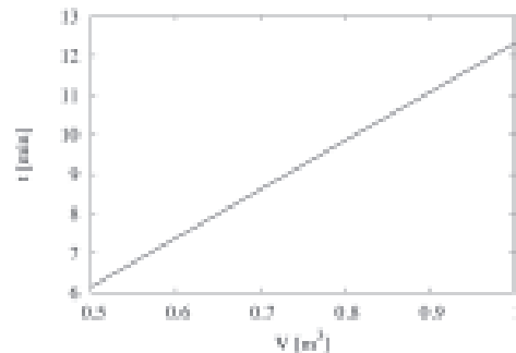
Kuva 4. Tiivistymisaika t kopin tilavuuden V funktiona.
