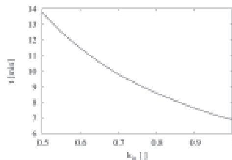
Kuva 5. Tiivistymisaika t vesihöyryn sisäänjäämiskertoimen k_{in} funktiona.
