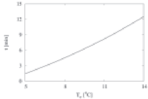
Kuva 3. Tiivistymisaika t kopin loppulämpötilan T_e funktiona.
