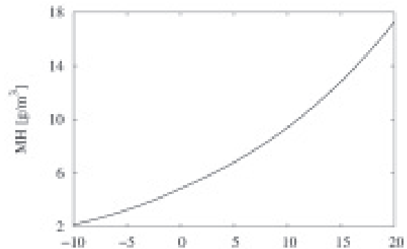
Kuva 1. Maksimikosteus lämpötilan funktiona.
